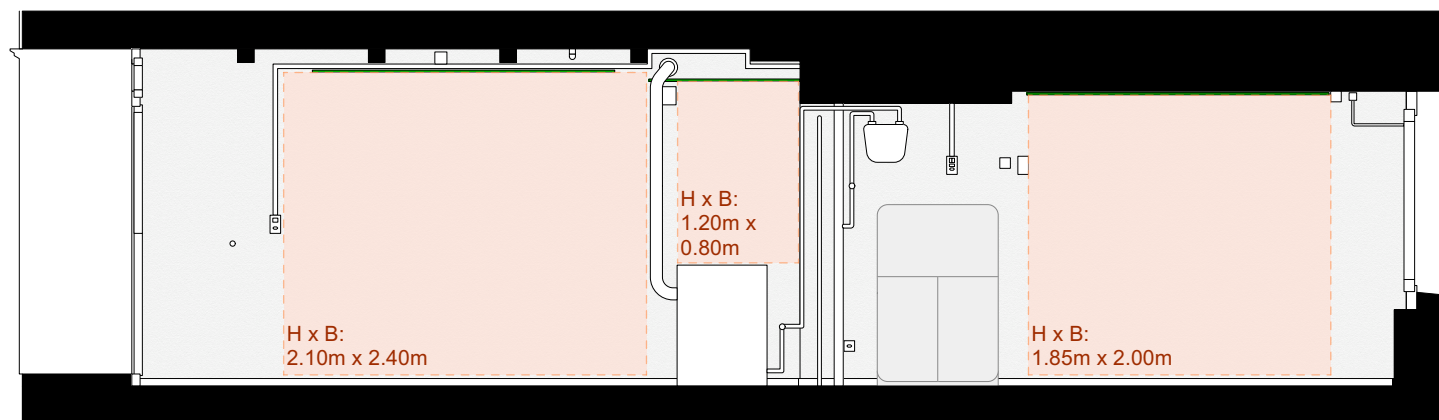
Ansicht Wand 1
