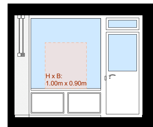
Ansicht Wand 4
