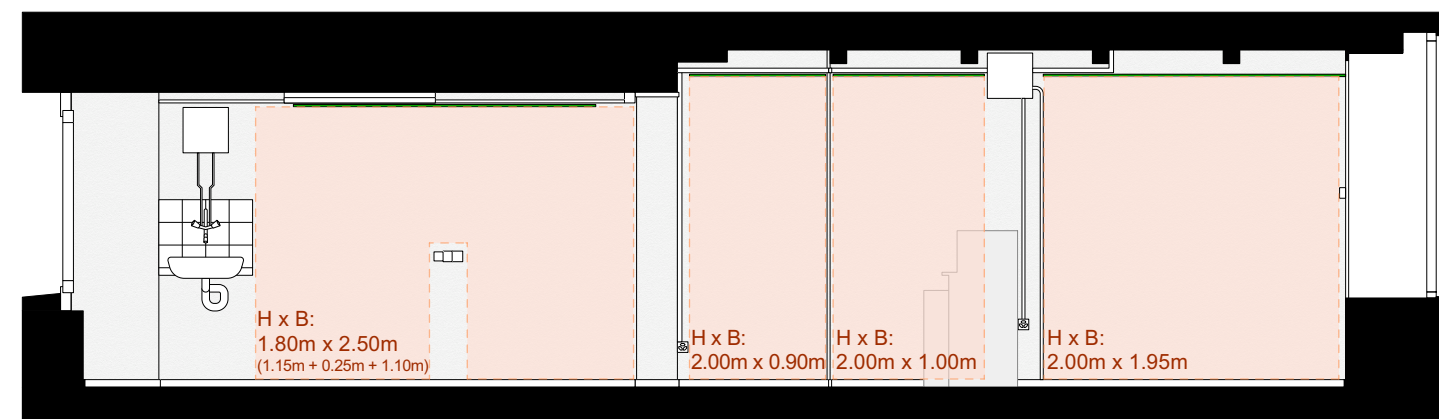
Ansicht Wand 3
